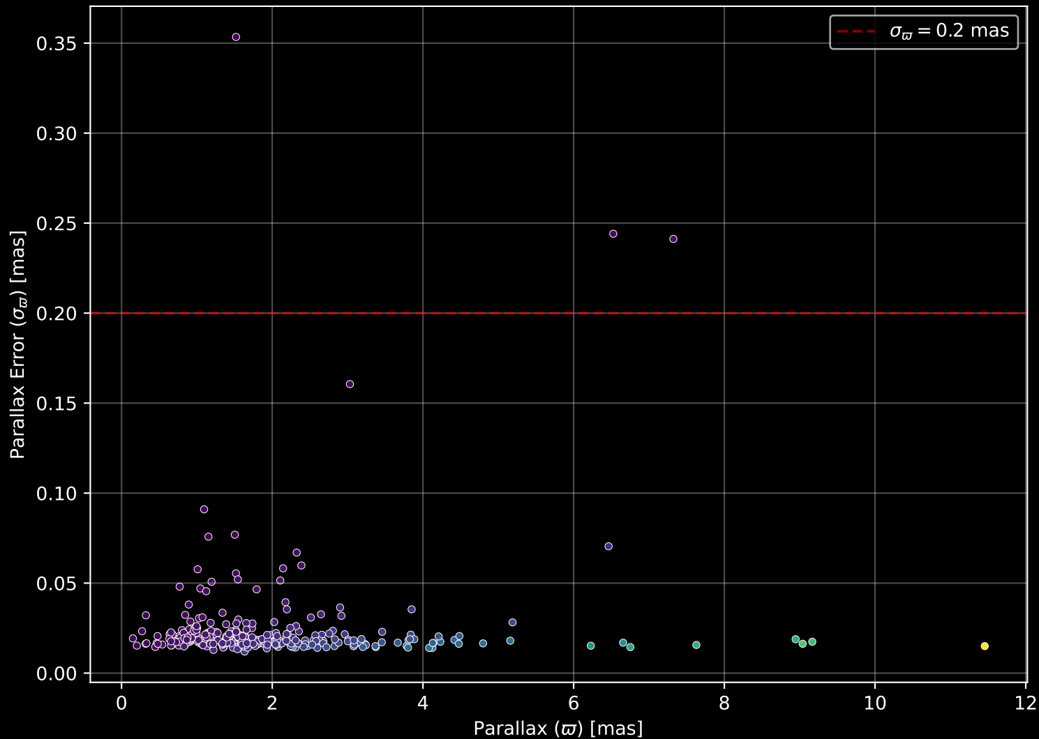
GALAH DR4 Field: [7029] Parallax Quality (n= 300)
