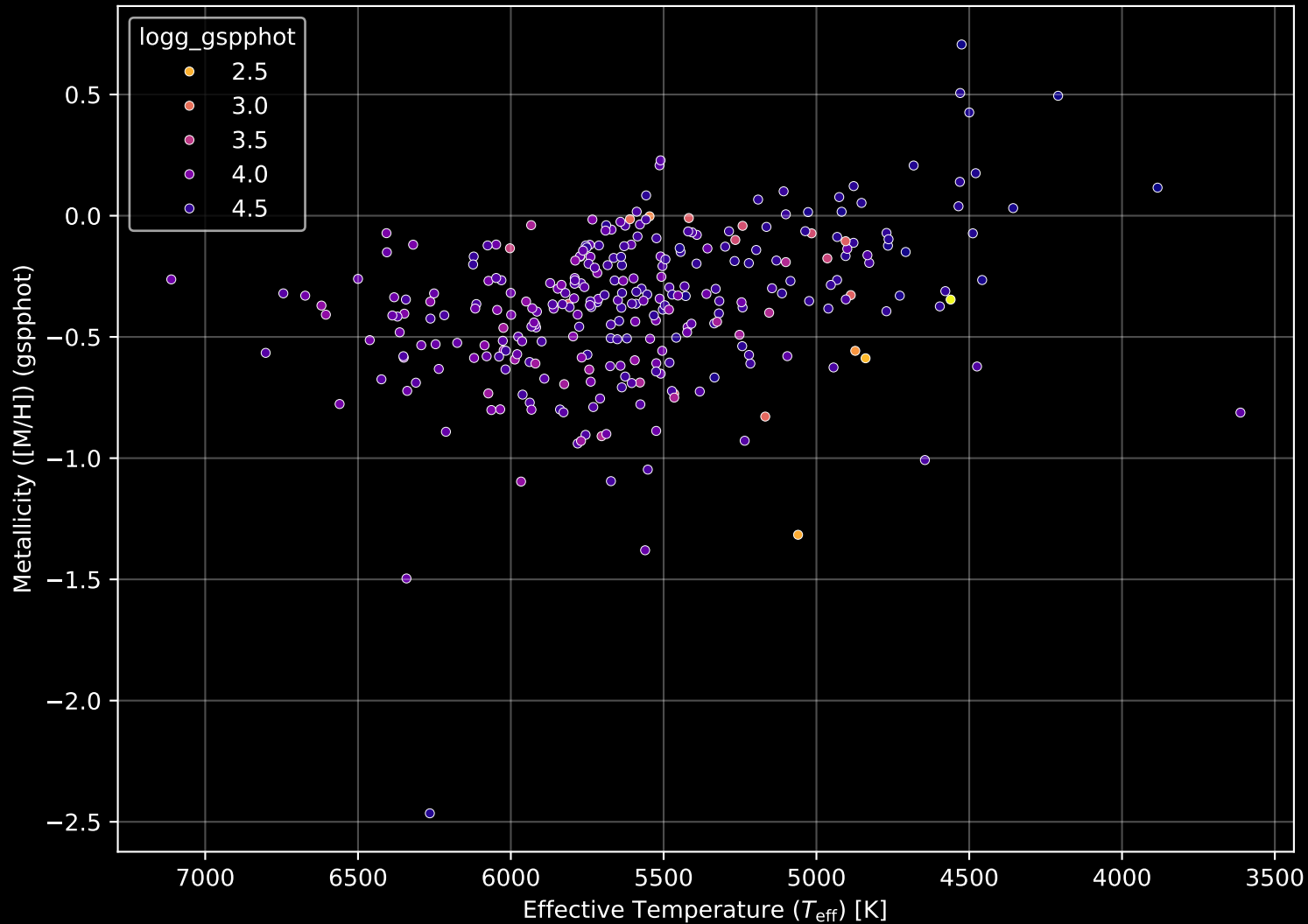
GALAH DR4 Field: [7029] Stellar Population Parameters (n= 300)
